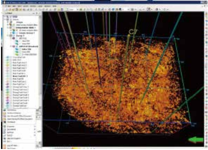
油藏地质建模
