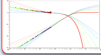
W 典型曲线分析
